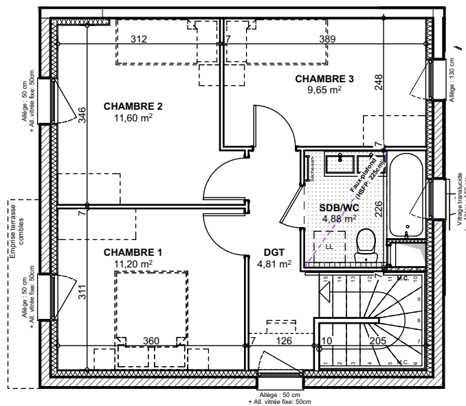
Plan du premier étage
