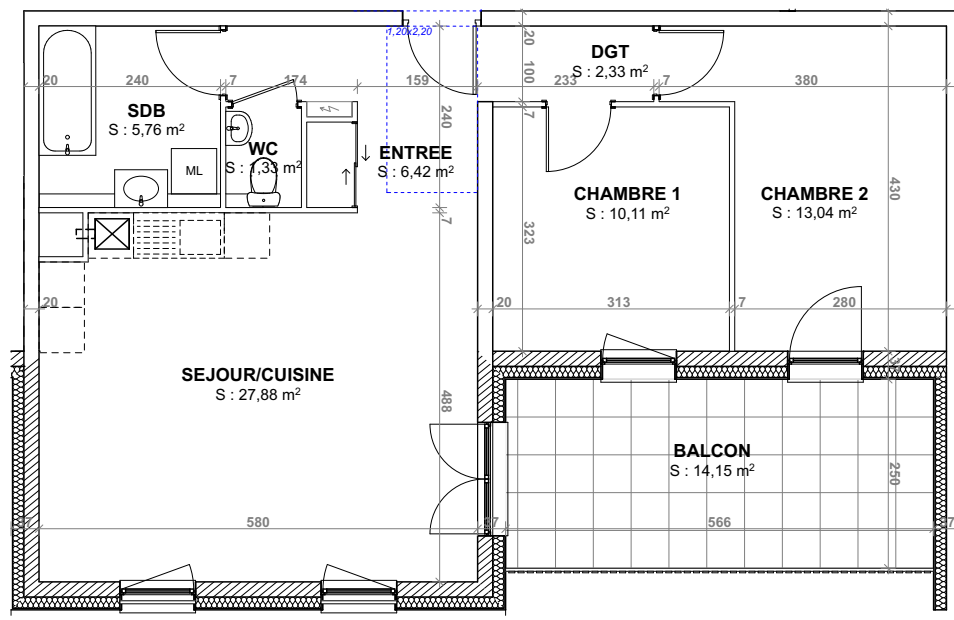
PLAN DU PREMIER ETAGE
