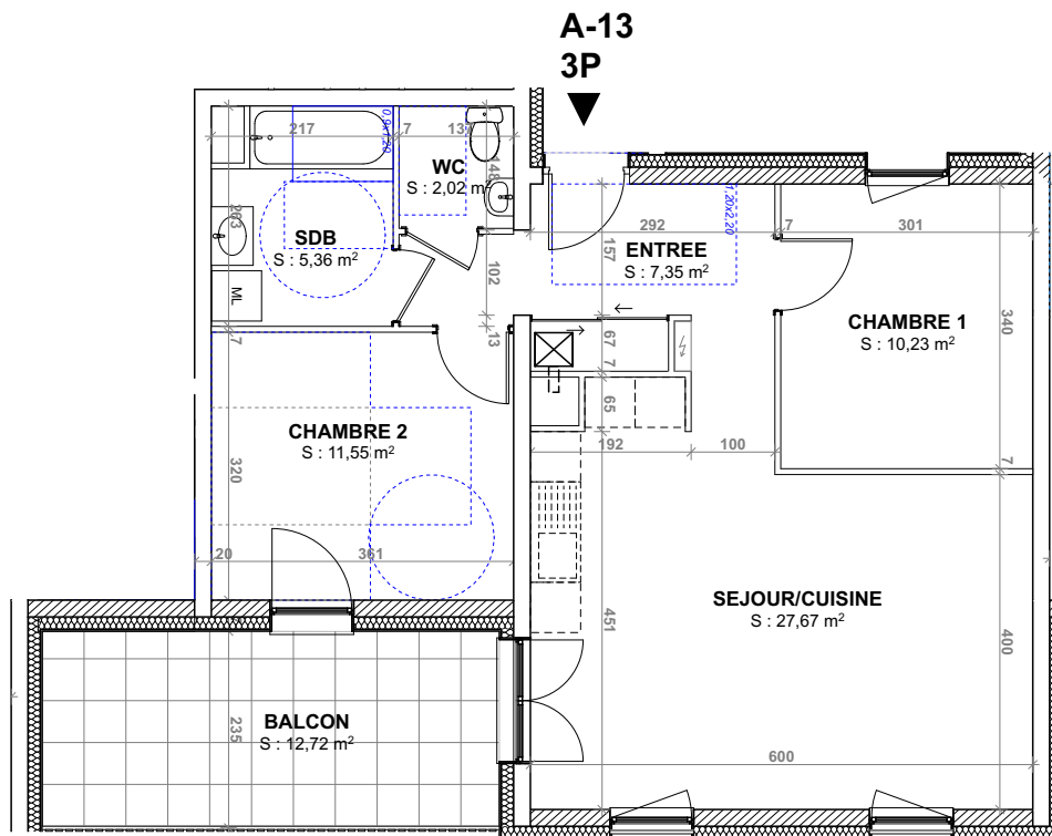
PLAN DU PREMIER ETAGE
