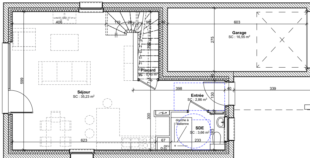
PLAN DU REZ-DE-CHAUSSEE
