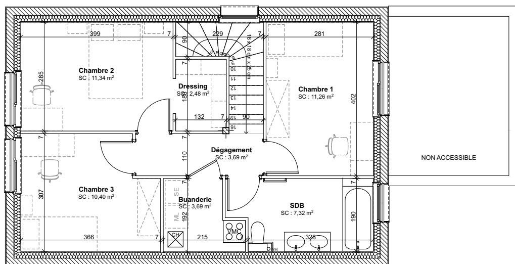
PLAN DU PREMIER ETAGE
