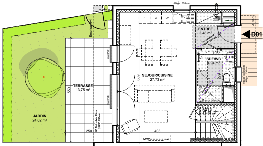
Plan du RDC
