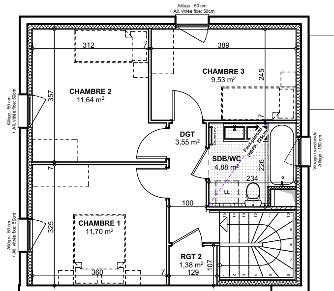
Plan du premier étage
