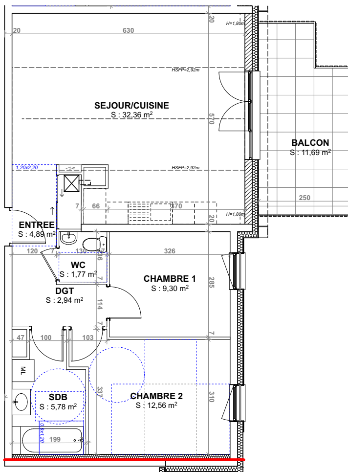
PLAN DU DEUXIEME ETAGE
