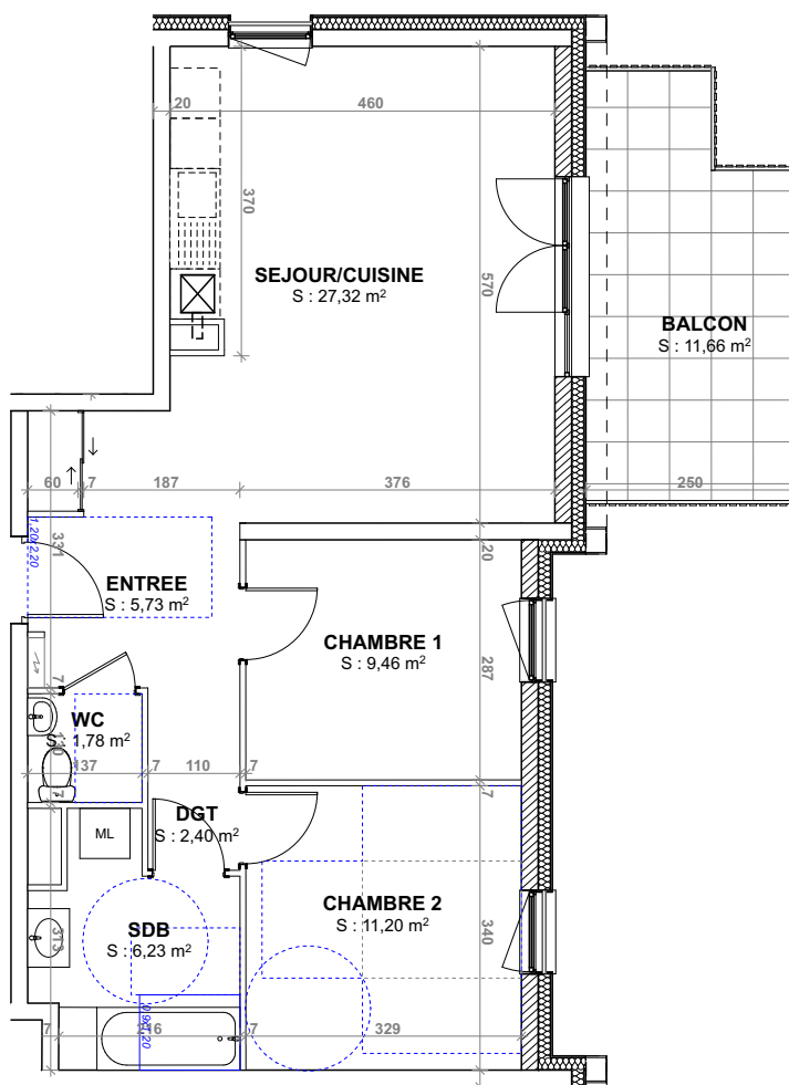
PLAN DU PREMIER ETAGE
