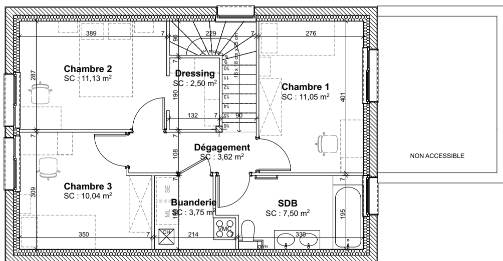
PLAN DU PREMIER ETAGE
